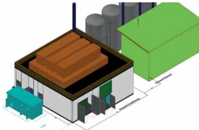
Isometrische Darstellung des Erweiterungsbaus des Heizwerks Am Erlberg (Grafik: EnergieAgentur Berghamer und Penzkofer)
